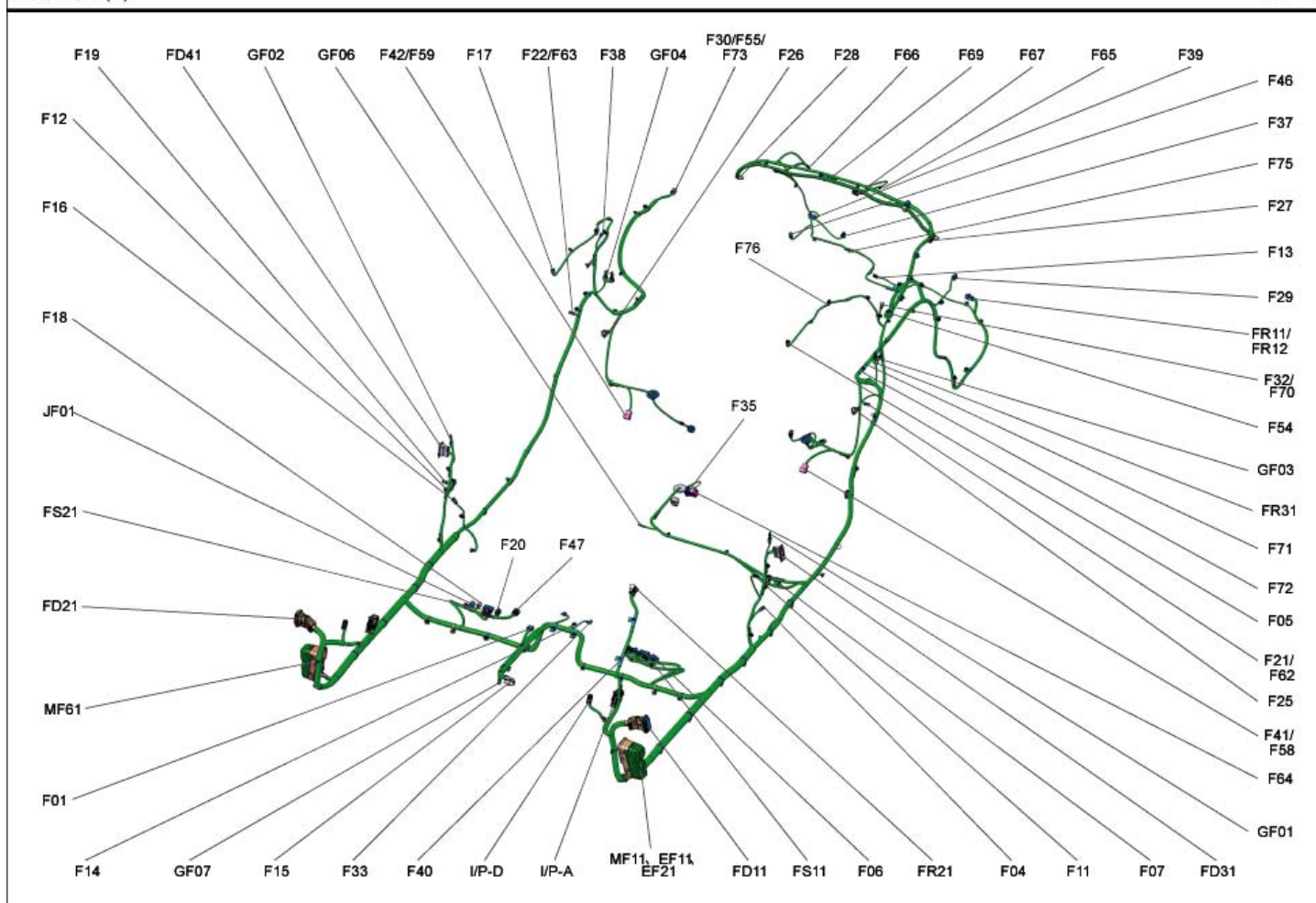
地板线束(1)
